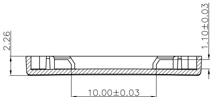
剖面 A-A
