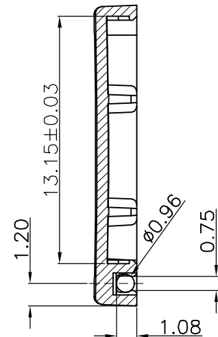
剖面 B-B
