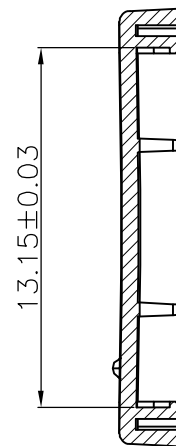
剖面 B-B
